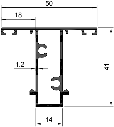
SECTION NO. - CA-1010 EST. WEIGHT - 0.642 KG./M.
